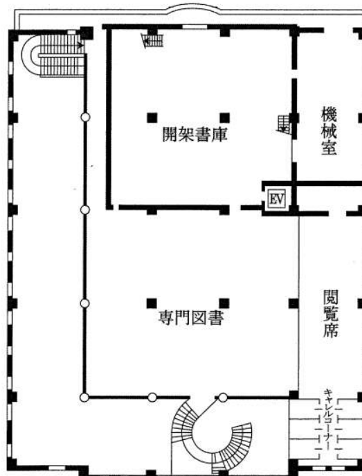
図書館 2 F
