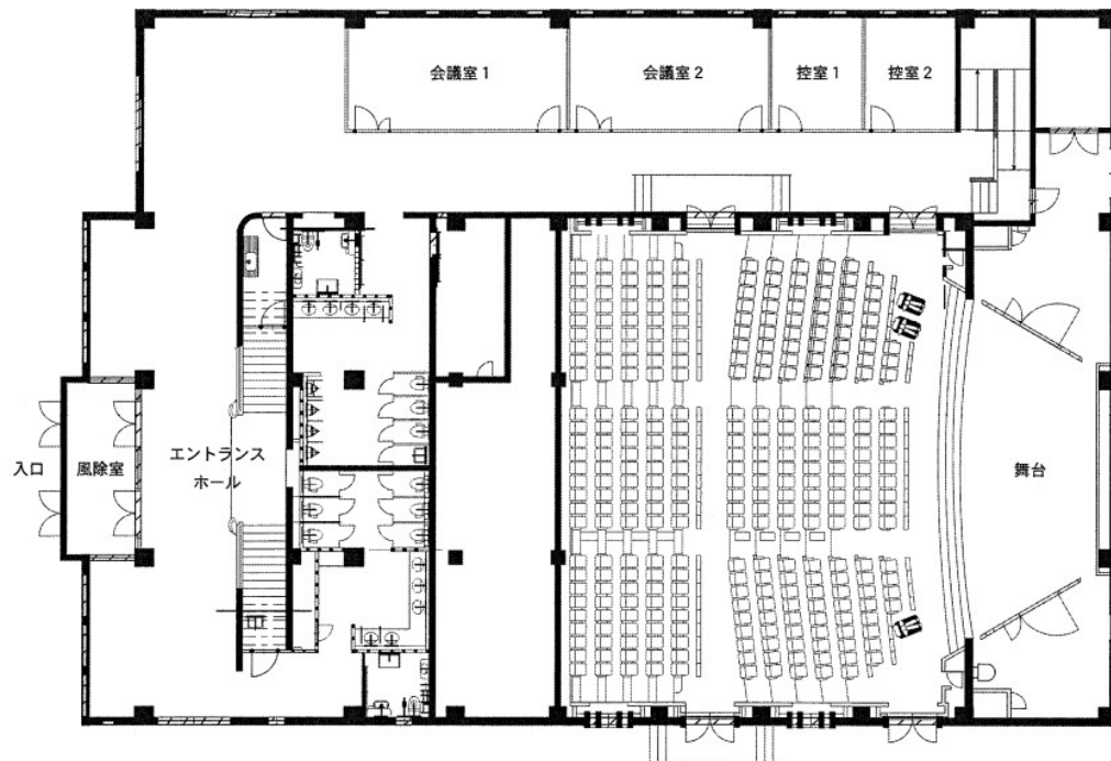
ホール 2 F
